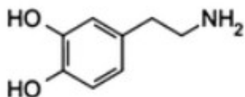
dopamine
