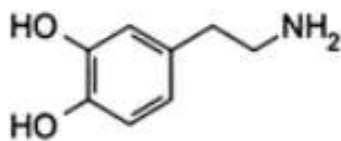
dopamine
